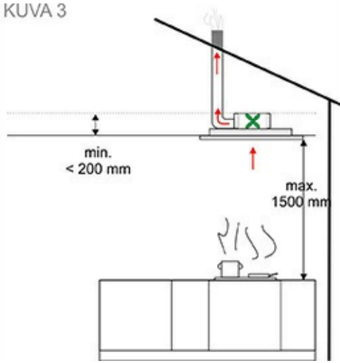
SLIM-moottori sijoitetaan suoraan kupuun
